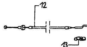
Kupplungszug
