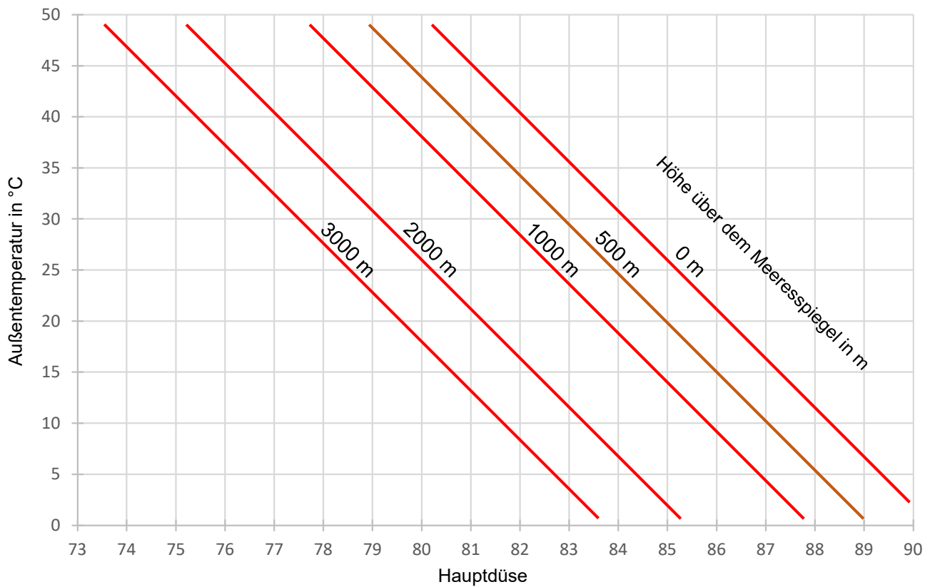
Hauptdüsen-Diagramm
