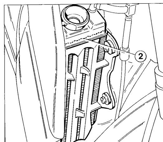
1) Tappo radiatore / Radiator plug / Bouchon radiateur / Kühlerverschluss / Tapa radiador 2) Livello liquido / Fluid level / Niveau liquide / Kühlflüssigkeitstand / Nivel liquido
