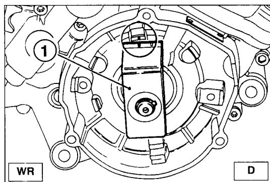
Anticipo/Spark advance/ Avance à l'allumage/ "a":
